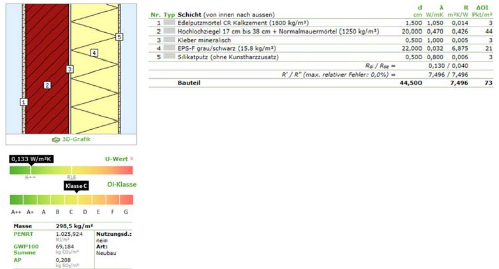
Abbildung 2: Darstellung OI Klasse (Quelle: www.baubook.at/eco2soft )
