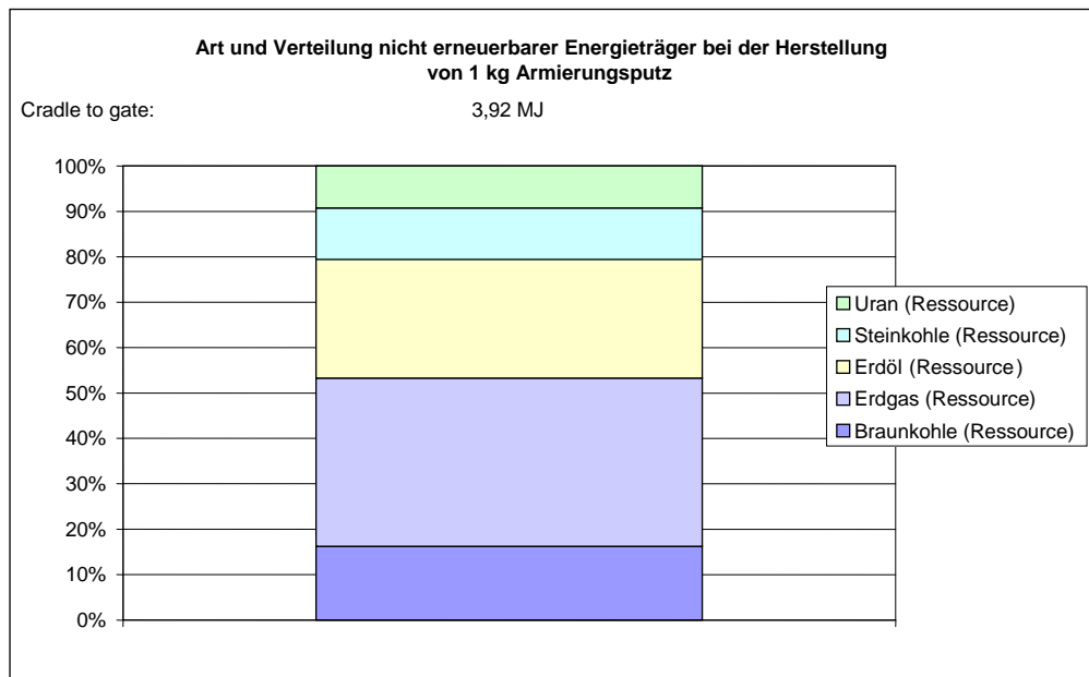
Abbildung 2: Art und Verteilung nicht erneuerbarer Energieträger bei der Herstellung von 1 kg Armierungsputz
