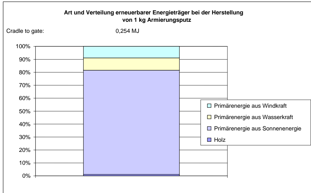
Abbildung 3: Art und Verteilung erneuerbarer Energieträger bei der Herstellung von 1 kg Armierungsputz
