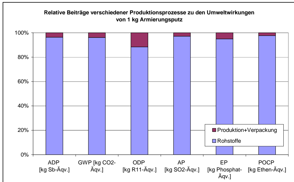
Abbildung 4: Relative Beiträge verschiedener Produktionsprozesse zu den Umweltwirkungen von 1 kg Armierungsputz
