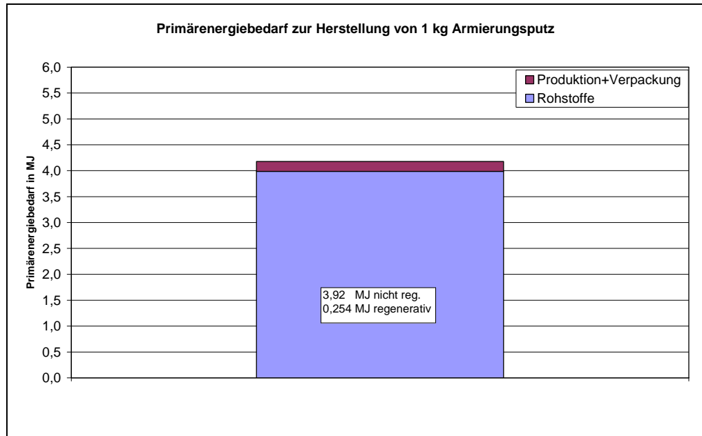
Abbildung 1: Primärenergiebedarf zur Herstellung von 1 kg Armierungsputz
