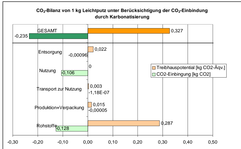
Abbildung 5: CO 2 -Bilanz von 1 kg Leichtputz unter Berücksichtigung der CO 2 -Einbindung durch Karbonatisierung
