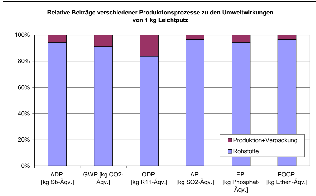
Abbildung 4: Relative Beiträge verschiedener Produktionsprozesse zu den Umweltwirkungen von 1 kg Leichtputz
