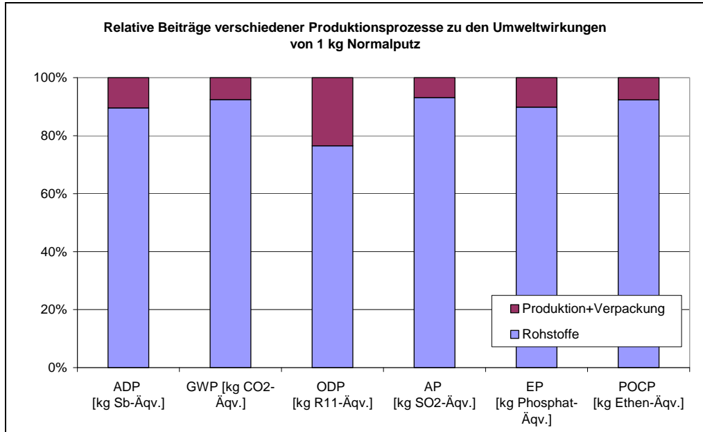
Abbildung 4: Relative Beiträge verschiedener Produktionsprozesse zu den Umweltwirkungen von 1 kg Normalputz
