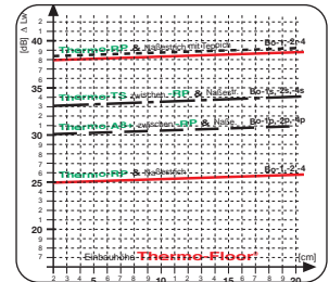
Trittschall-Richtwerte (Massivdecke)
