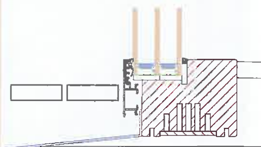
Festverglasung: Fenster unten
