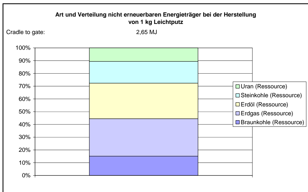
Abbildung 2: Art und Verteilung nicht erneuerbarer Energieträger bei der Herstellung von 1 kg Leichtputz
