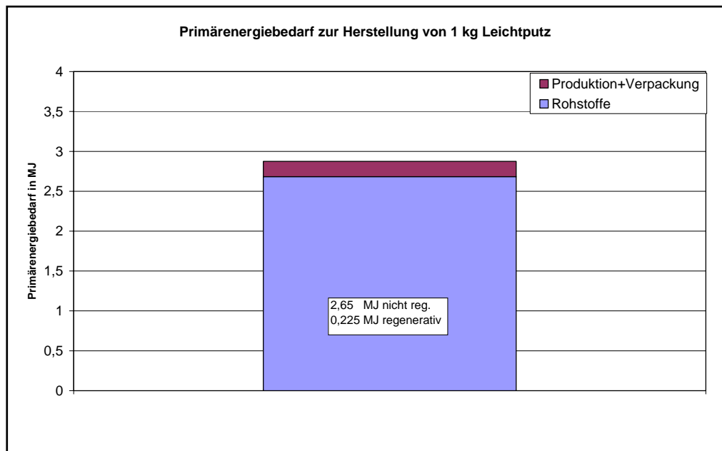
Abbildung 1: Primärenergiebedarf zur Herstellung von 1 kg Leichtputz
