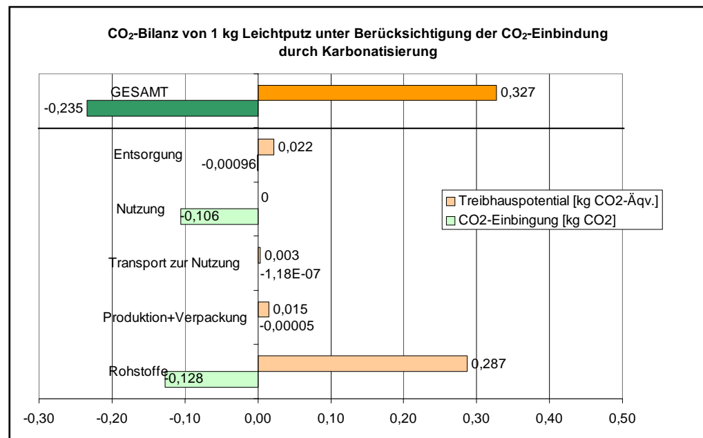
Abbildung 5: CO 2 -Bilanz von 1 kg Leichtputz unter Berücksichtigung der CO 2 -Einbindung durch Karbonatisierung
