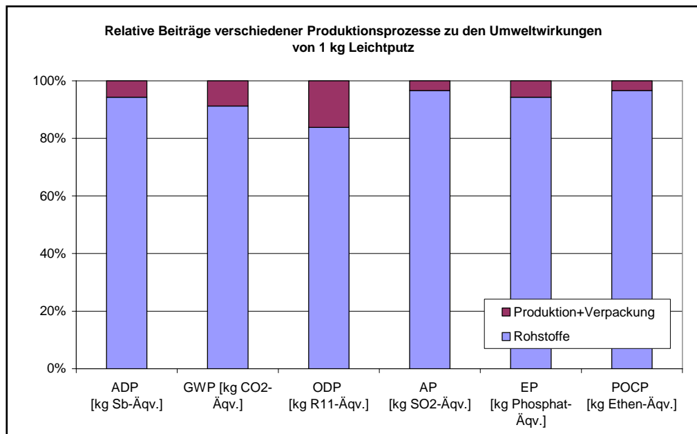
Abbildung 4: Relative Beiträge verschiedener Produktionsprozesse zu den Umweltwirkungen von 1 kg Leichtputz
