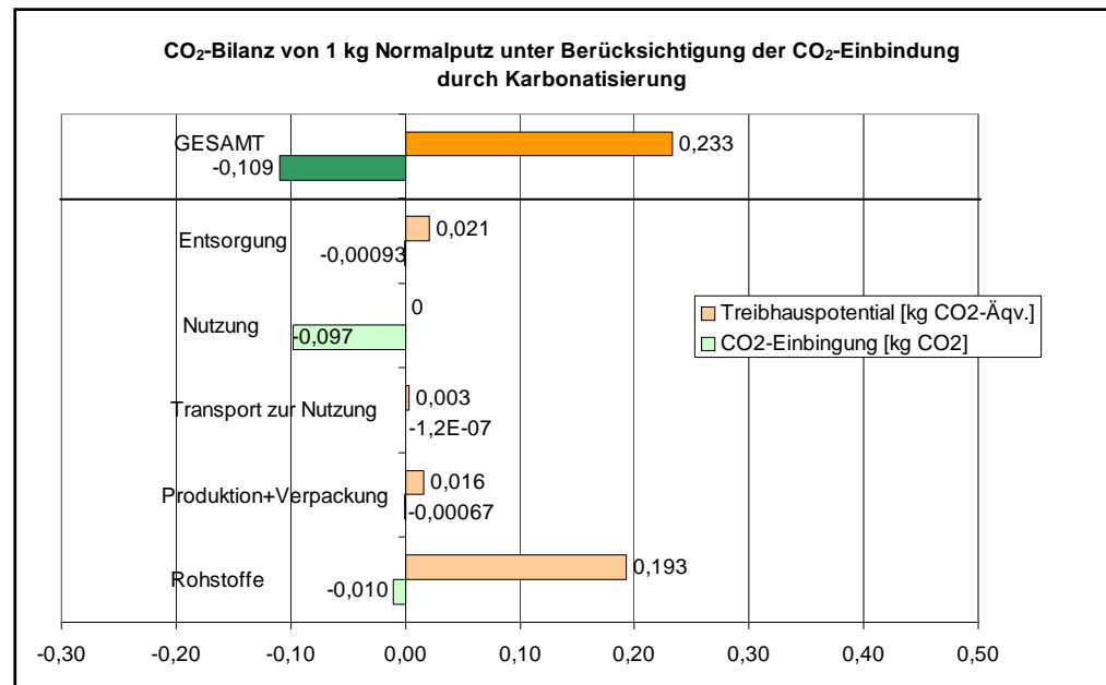
Abbildung 5: CO 2 -Bilanz von 1 kg Normalputz unter Berücksichtigung der CO 2 -Einbindung durch Karbonatisierung
