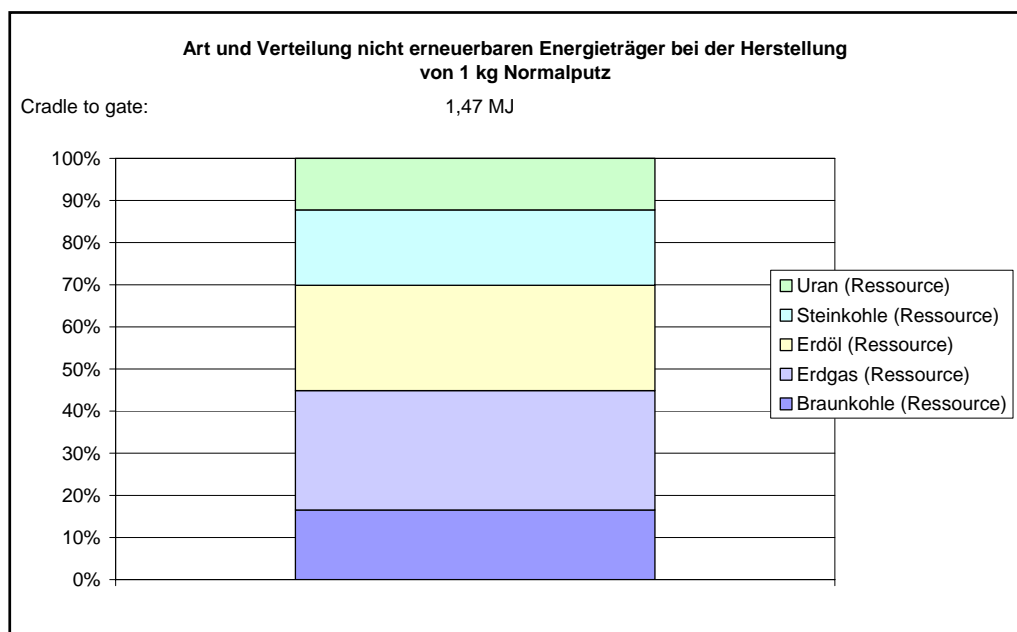
Abbildung 2: Art und Verteilung nicht erneuerbarer Energieträger bei der Herstellung von 1 kg Normalputz
