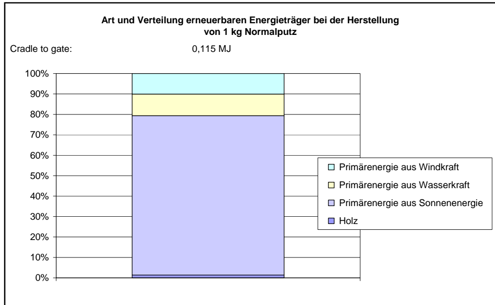
Abbildung 3: Art und Verteilung erneuerbarer Energieträger bei der Herstellung von 1 kg Normalputz
