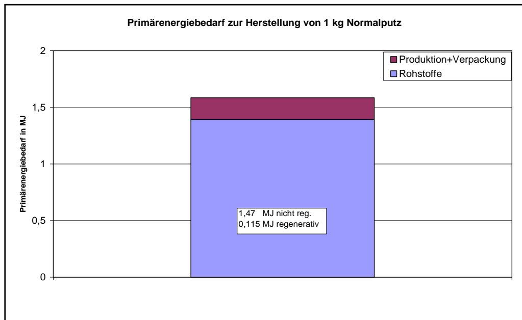
Abbildung 1: Primärenergiebedarf zur Herstellung von 1 kg Normalputz
