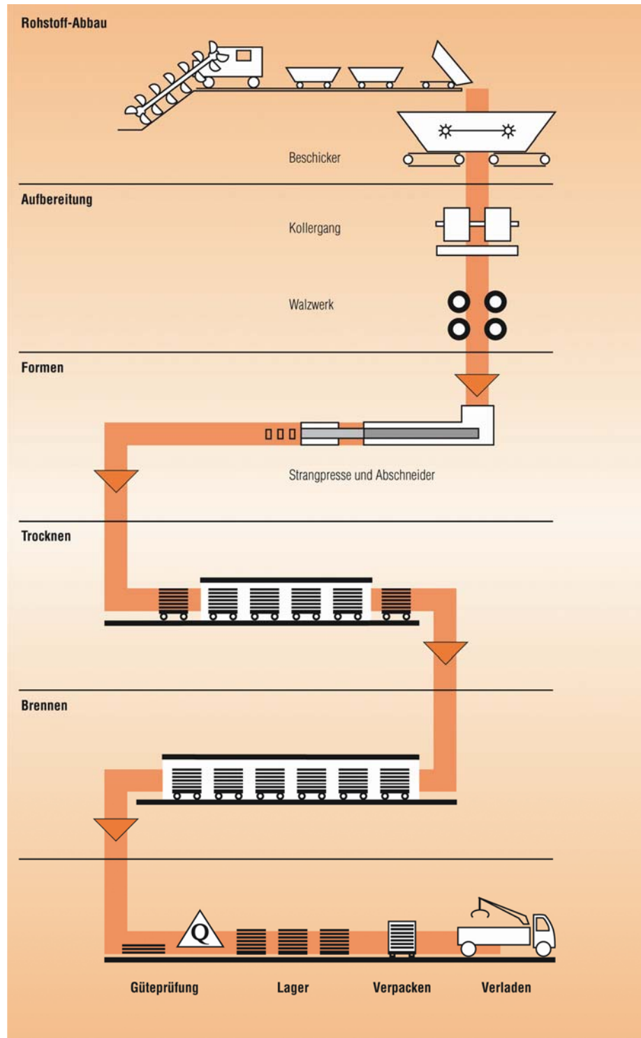
Abbildung 1: Schematische Darstellung der Ziegelstein-Produktion
