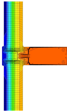
Isothermengrafik
