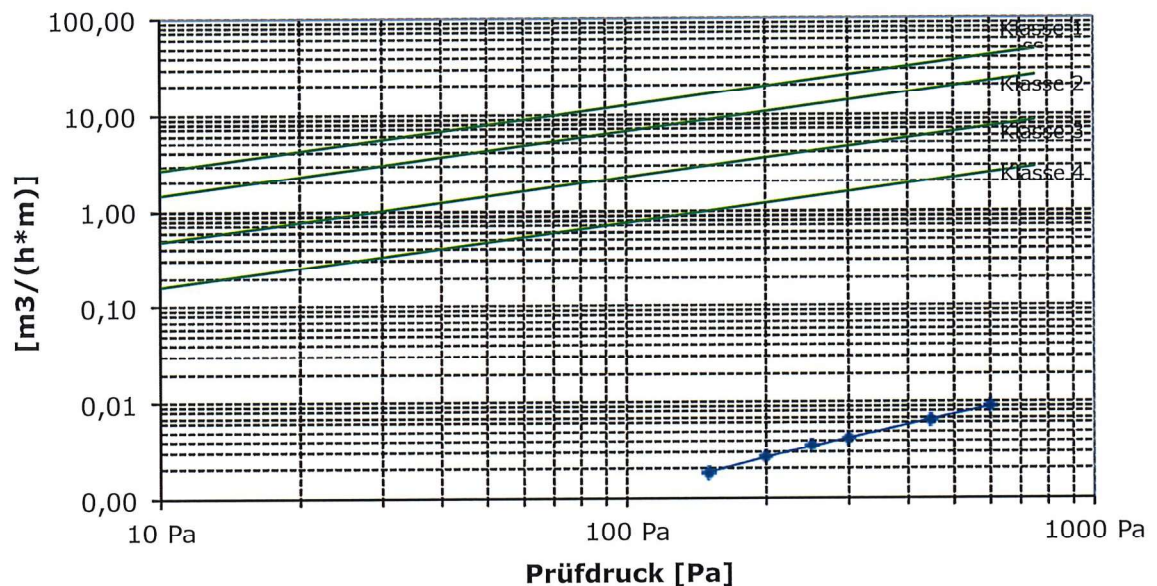
Diagramm 1: Grafische Darstellung der längenbezogenen Luftdurchlässigkeitsklassen (ohne Abzug der Prüfstandundichtigkeit)
