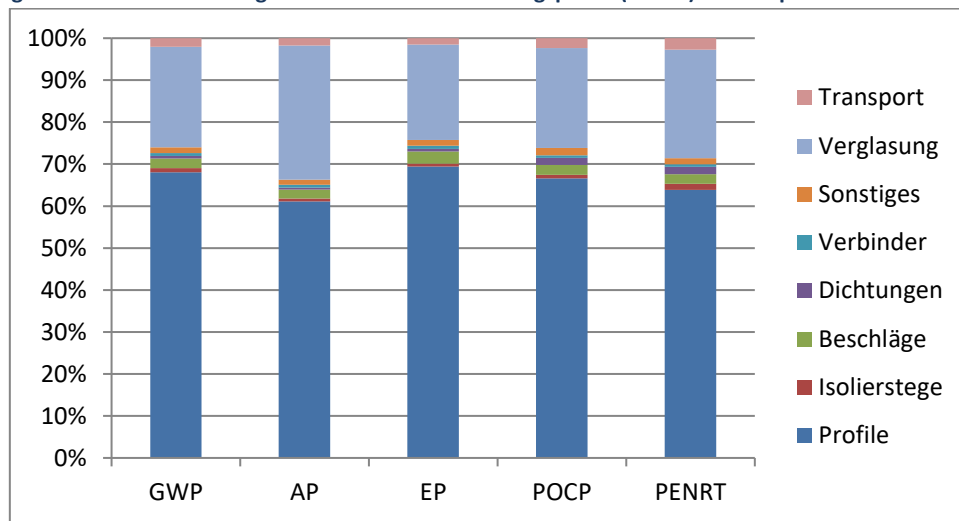
Abbildung 3: Anteile der Belastungen während der Herstellungsphase (A1-A3) am Beispiel des Produkts FWS 60 CV
