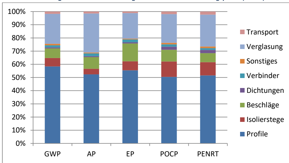
Abbildung 3: Anteile der Belastungen während der Herstellungsphase (A1-A3)
